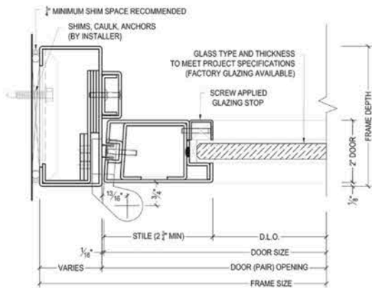
JAMB / PIVOT STILE
