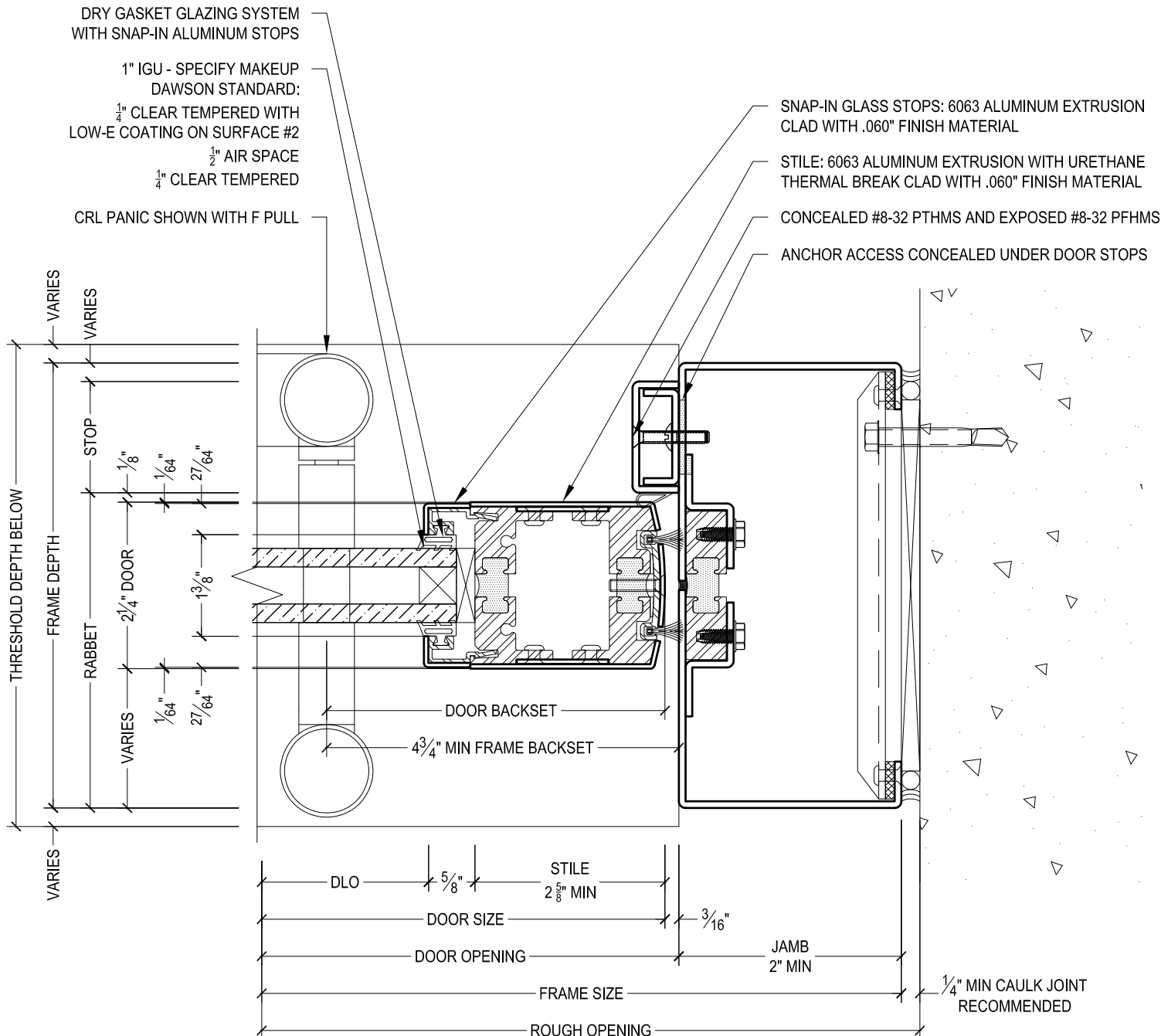
6 LOCK STILE Scale: 1:2
